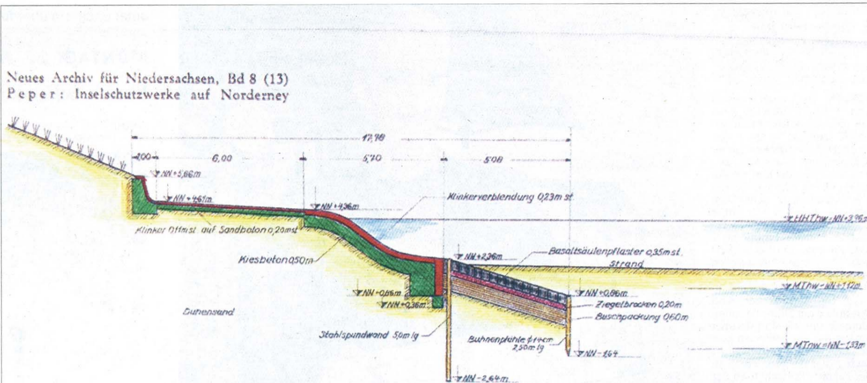
Abb. 4 Querschnitt durch die Strandschutzmauer von Bühne H 1 bis L 1
