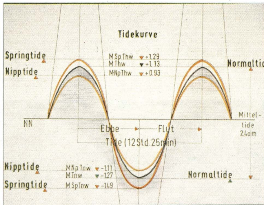
Reguläre Tidekurve.
