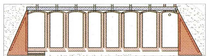
Wasserreservoir „Georgshöhe“ Rekonstruktionszeichnung: Bernd Röben, Norderney
