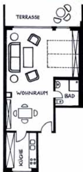
PARTERRE
