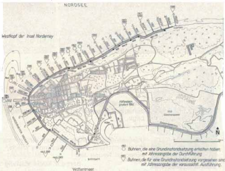
Plan der Inselfschutzwerke rund um den Westkopf 1985
