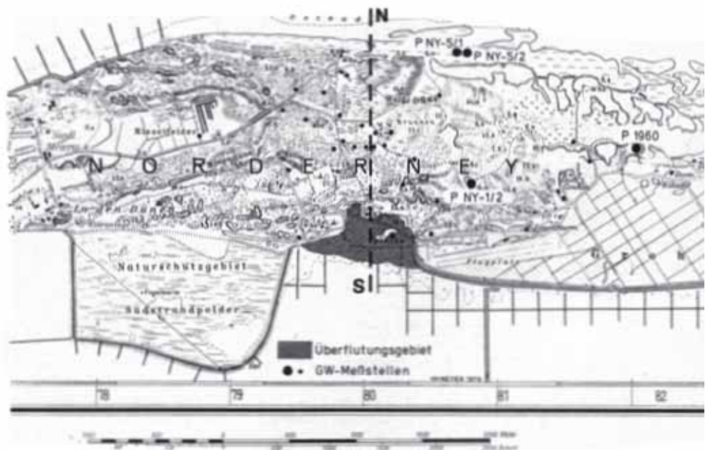
Grundwasser-Meßstation und Lageplan des Meßstellennetzes auf Norderney. Installiert sind 50 Meßeinrichtungen, davon sind 10 mit Schreibgeräten ausgestattet.
