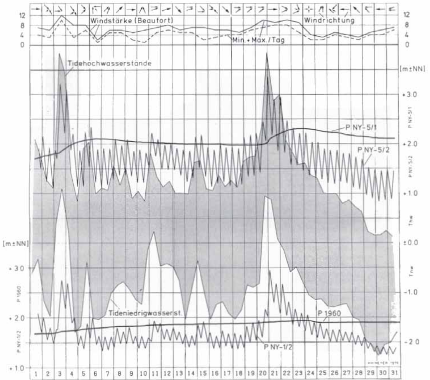
Wasserstände im Januar 1976 auf Norderney
