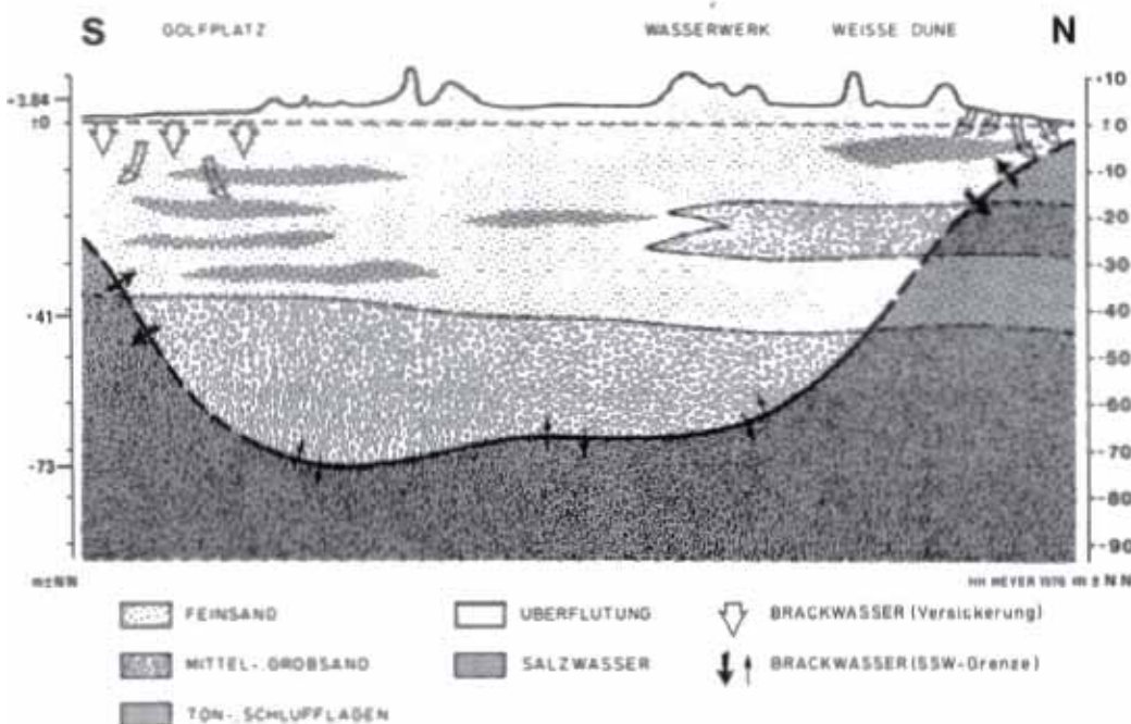
Schnitt durch die Süßwasserlinse im Bereich des Wasserwerkes „Weiße Düne“
