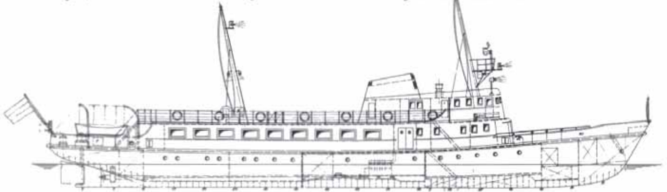
Im maßstabgerechten Vergleich der Schiffsrisse der alten und modernisierten „Frisia III“ sieht man deutlich die baulichen Veränderungen, wobei insbesondere die neue gestreckte Form des Schiffsrumpfes und die Erweiterung der Decks auffallen.
